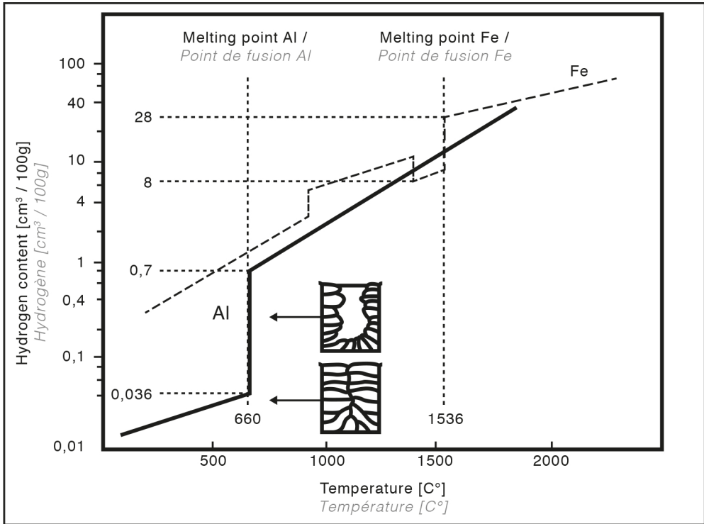
Solubility of hydrogen in aluminium and iron / Solubilité de l'hydrogène dans l'aluminium et l'acier
